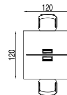
Ensemble 2 positions L.120cm P.120cm H.74cm Séparation H.35cm
