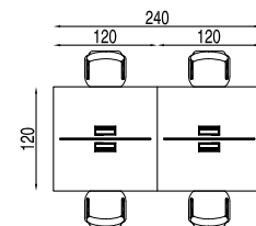
Ensemble 4 positions L.240cm P.120cm H.74cm Séparation : H.35cm
